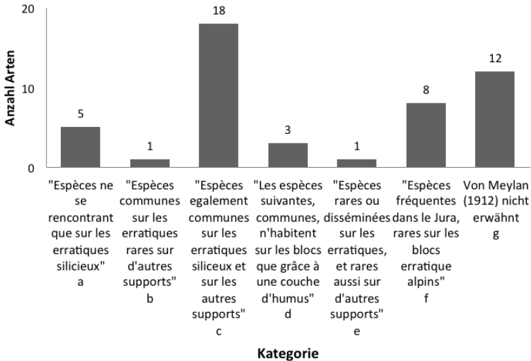
Abb. 3 Klassen, nach denen Meylan (1912) Moose im Jura gemäss ihrer Spezifität für silikatische Findlinge einteilte und ihre Codierung (Tab. 1).
